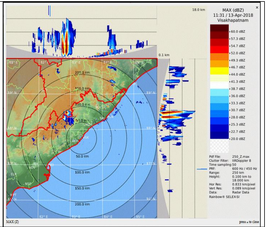
Radar Composite at 1702 IST of the Day
