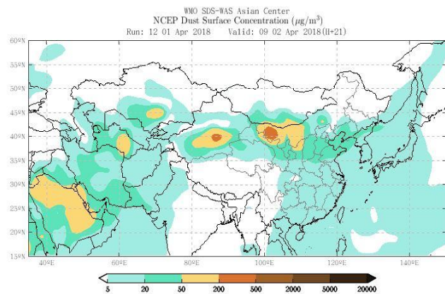
Dust AOD Forecast
