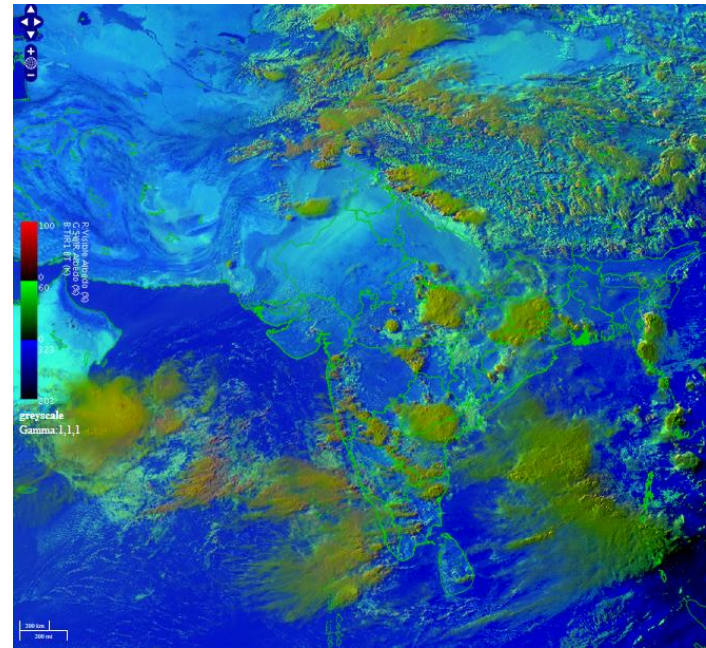
RAPID RGB Satellite Imagery at 1700 hrs IST of today
