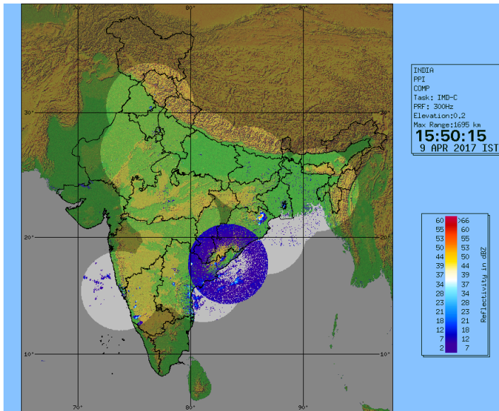
DWR Composite at 1550 hrs IST of today
