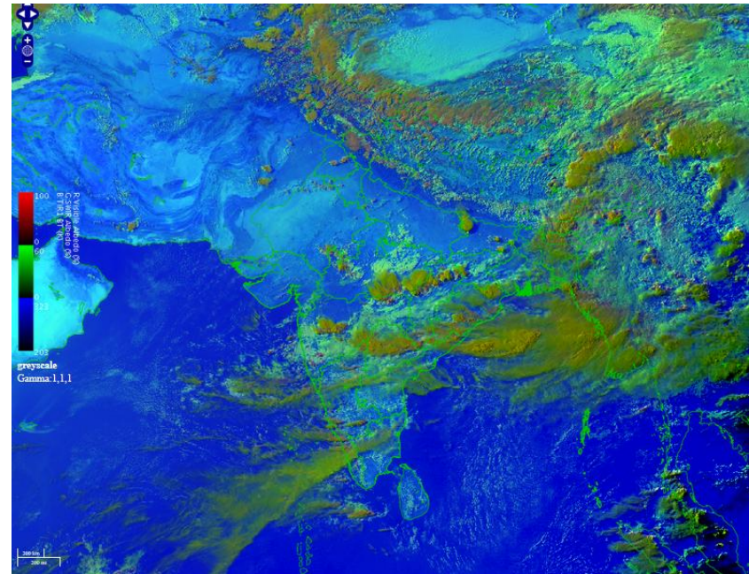
RAPID RGB Satellite Imagery at 1630 hrs IST of today
