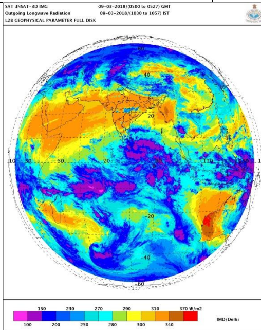
INSAT 3D OLR Imagery (1000-1027 IST today)
