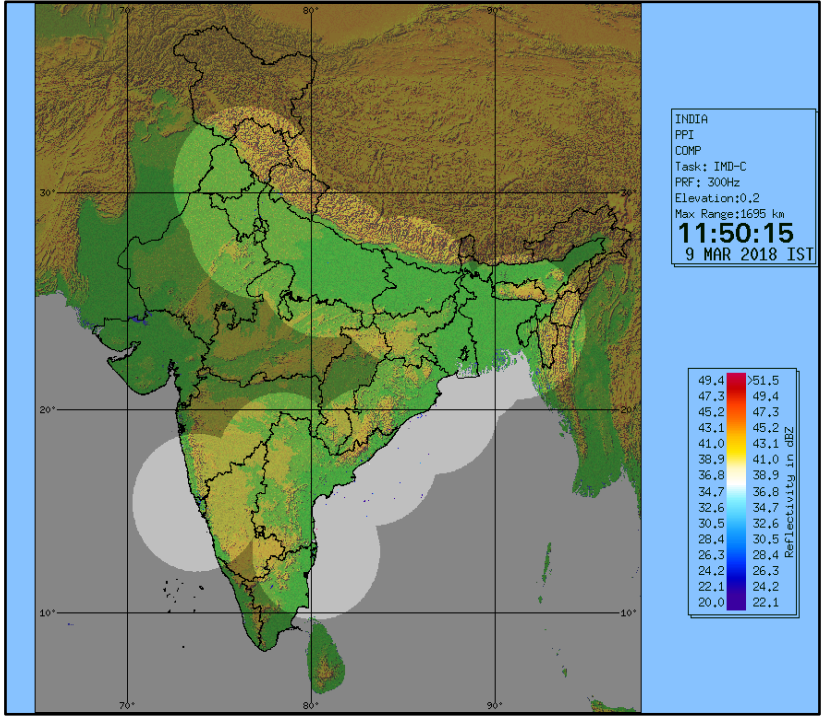
DWR Composite at 1150 IST of the Day
