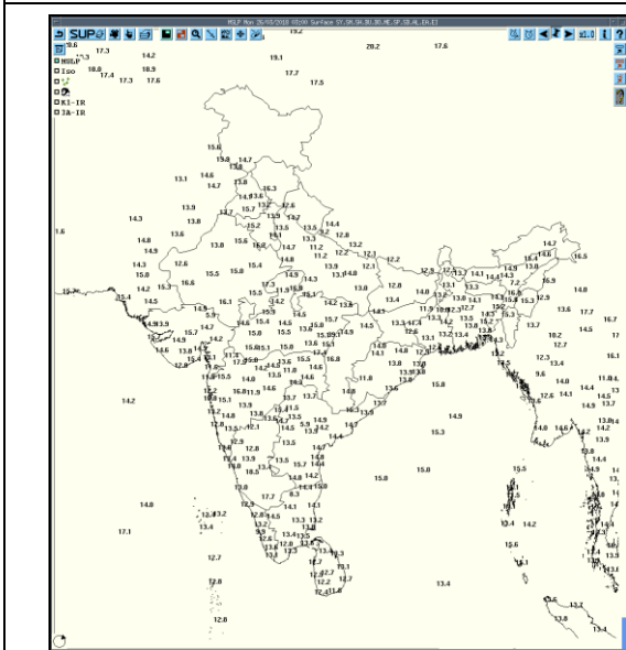
MSLP
