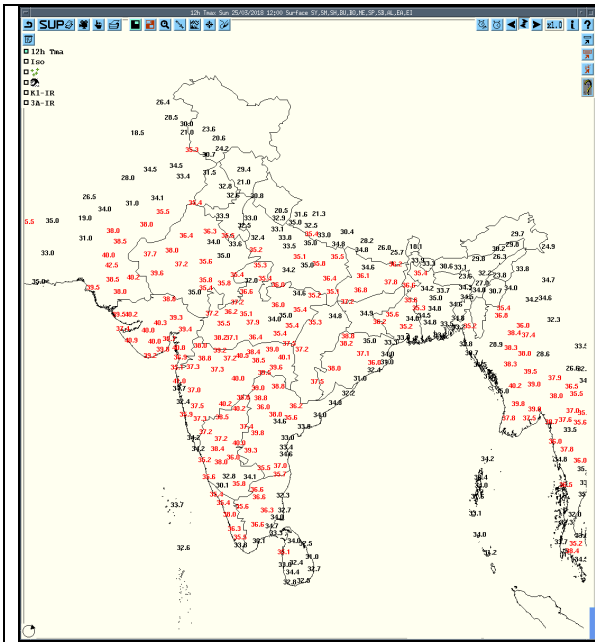
Tmax
