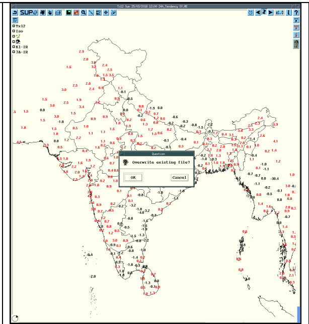
Tendency Tmax
