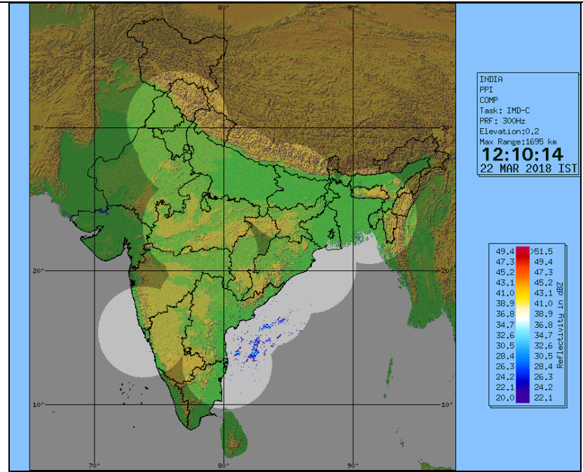
DWR Composite at 1210 IST of the Day
