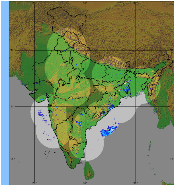
DWR composite at 1640 hrs IST
