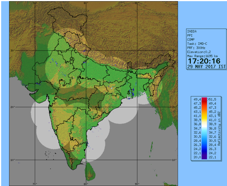
DWR Composite at 1720 hrs IST of today
