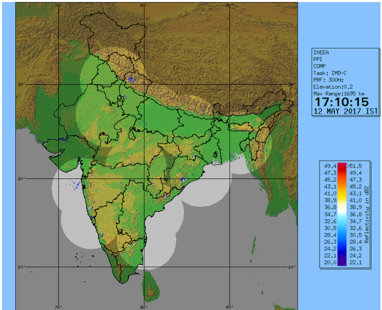
DWR Composite at 1710hrs IST of today
