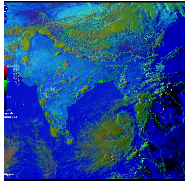
RAPID RGB Image of INSAT-3D at 1630 hrs IST of today
