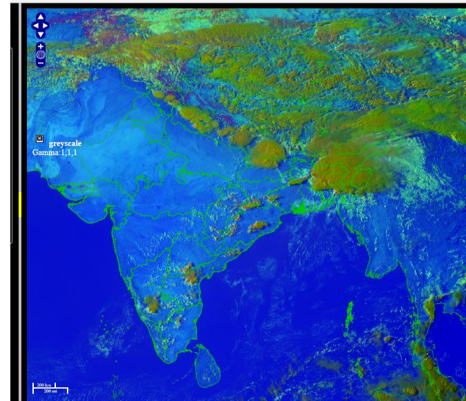
RAPID RGB Image of INSAT 3D at 1600 hrs IST of today
