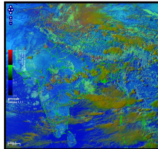
RAPID RGB Satellite Imagery at 1600 hrs IST of today
